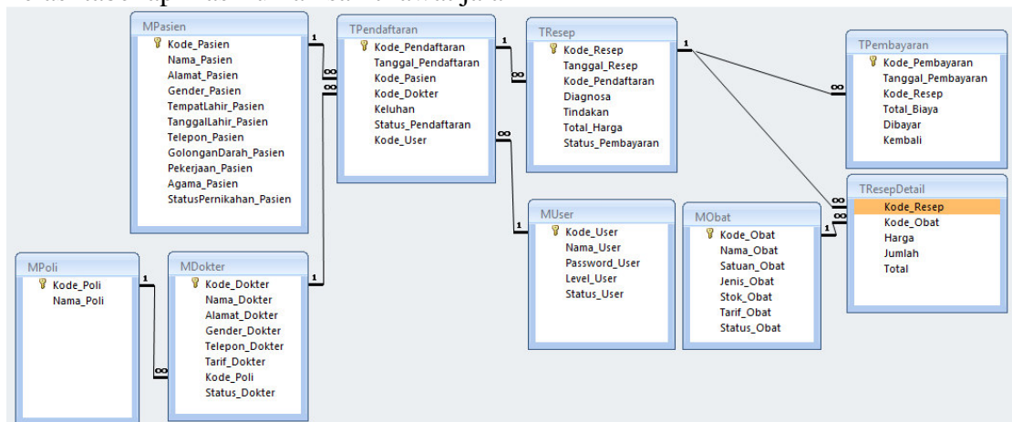
Relasi tabel aplikasi rumah sakit rawat jalan
